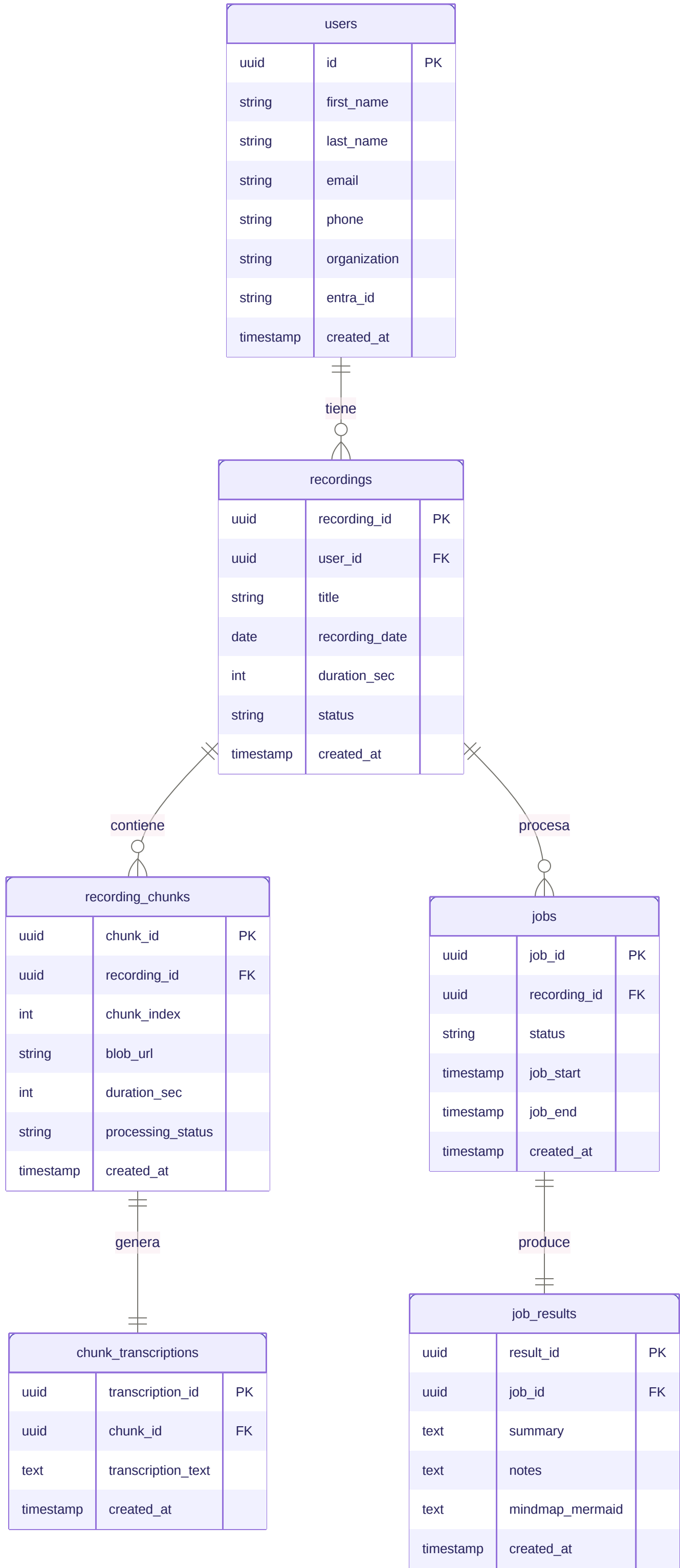
Database schema
